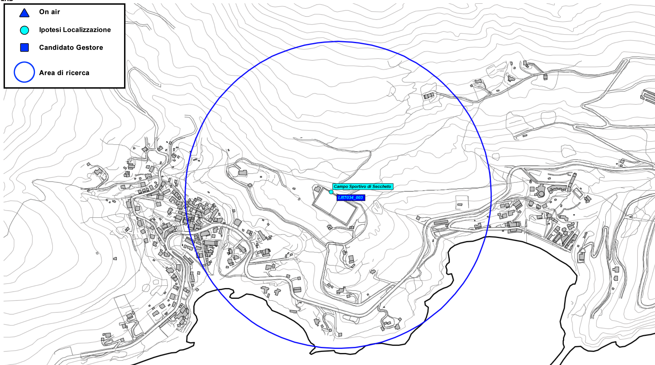
Fig. 24 Dettaglio piano di rete – Gestore ILIAD
