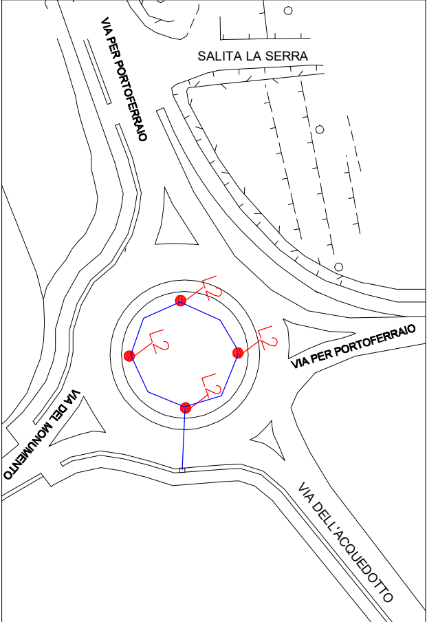
Schema impianto di progetto - Rotatoria La Serra
