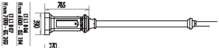
Modello Lampione Artistico - Sant'Illario
