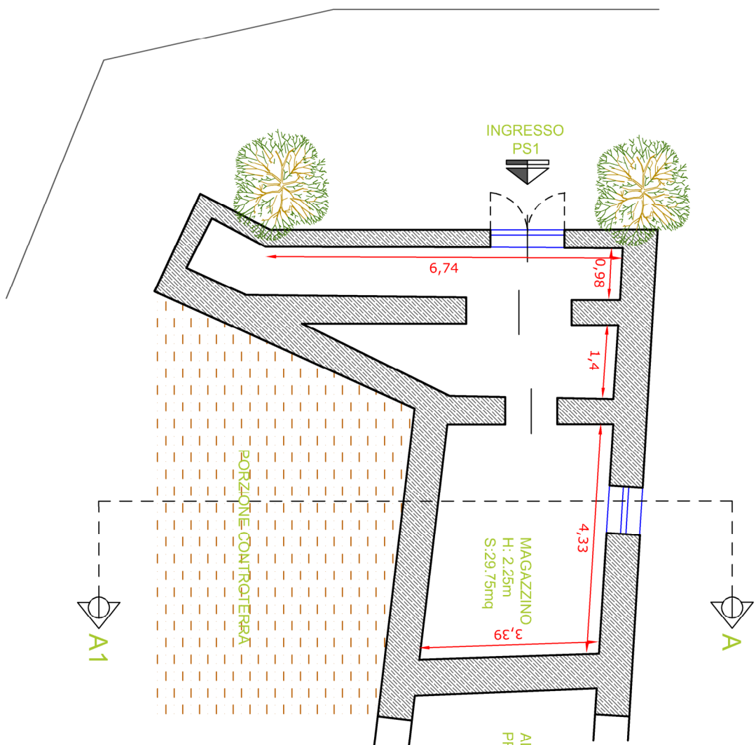
PIANO SEMINTERRATO (S1) - STATO PROGETTUALE SCALA 1:100
