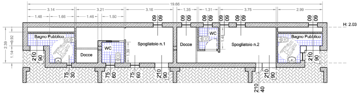
PIANTA SOTTO TRIBUNE STATO DI PROGETTO Scala 1:100
