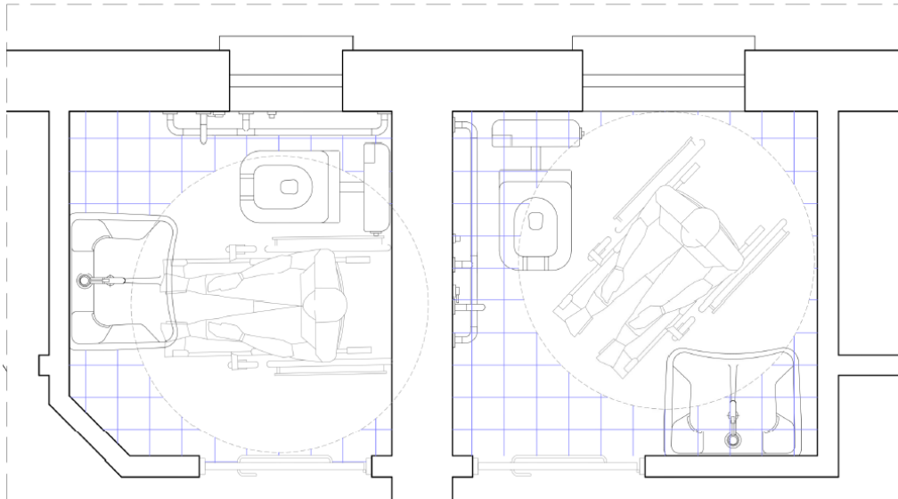
Particolari Bagno Disabili
