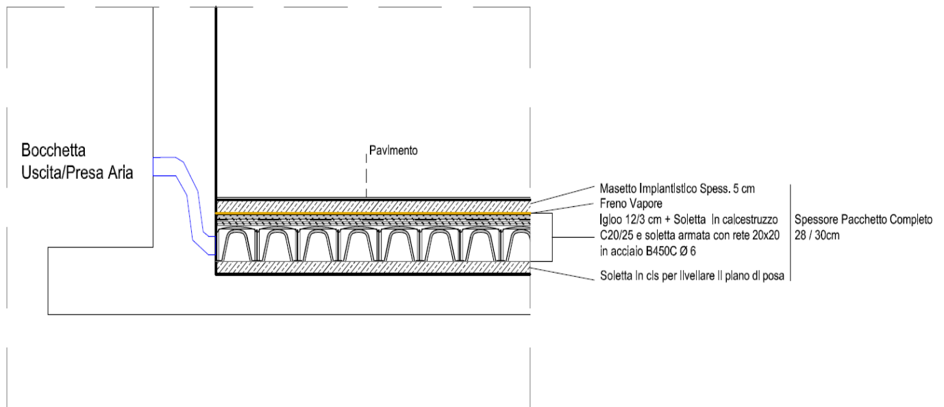
Particolare costruttivo Solaio Areato con Igloo
