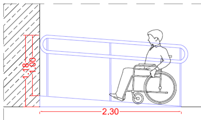
Particolari Rampa di Accesso
