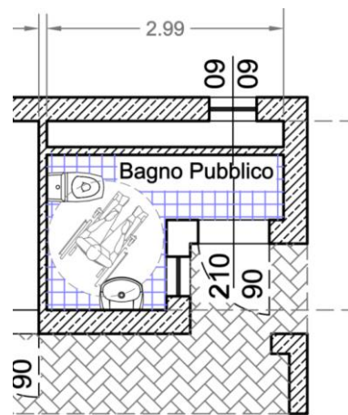
Particolari Nuovo Bagno Disabili
