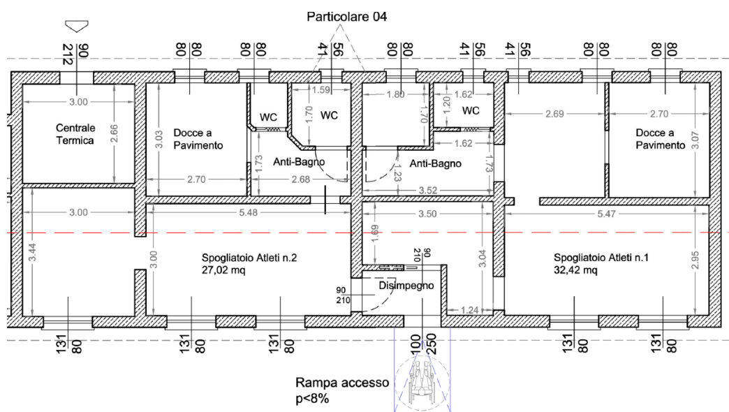
Estratto Tav_02: Spogliatoi Squadre
