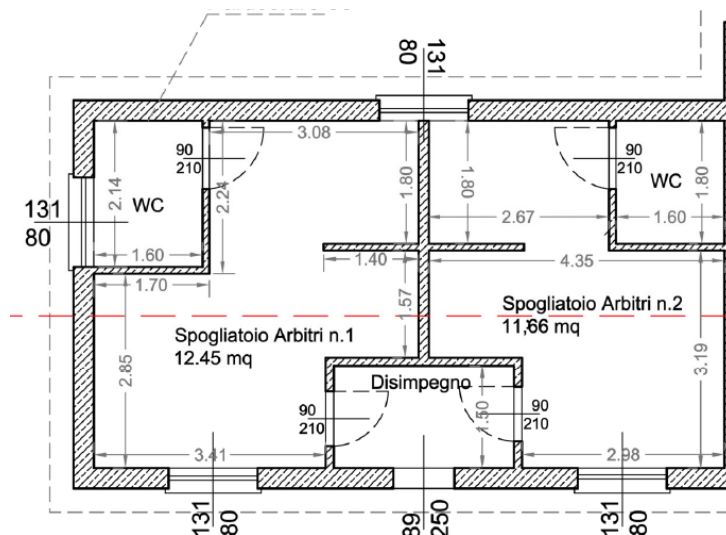
Estratto Tav_02: Spogliatoi Arbitri
